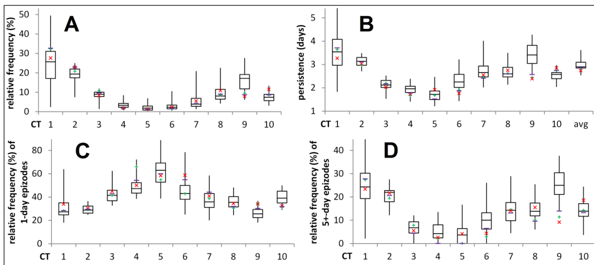
Obr. 3. Vlastnosti cirkulačních typů zobrazených na obr. 2. A relativní četnost, B perzistence, C relativní četnost 1denních epizod, D relativní četnost epizod s délkou trvání 5 a více dnů. Boxploty zobrazují kvartily, maximum a minimum ensmbu 33 GCMs, barevné symboly pak hodnoty pro reanalýzy (modře ERA-40, zeleně NCEP/NCAR, červeně 20CRv2).
