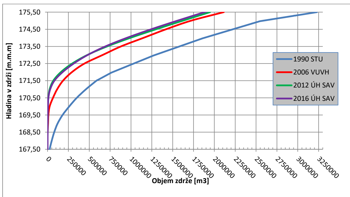
Obr. 7. Vývoj objemu VD Veľké Kozmálovce- vplyv zanášania Fig. 7. Trends in the volume of the WD Veľké Kozmálovce - impact of sediment fouling
